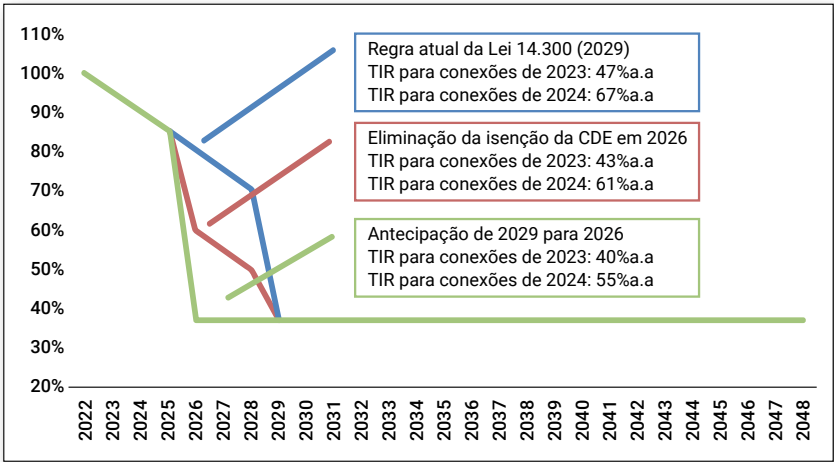
Figura 10 – Percentual da tarifa de aplicação ( netmetering ) com efeito na rentabilidade do empreendimento, conforme o cenário de antecipação dos prazos da Art 27º da Lei 14.300/22
