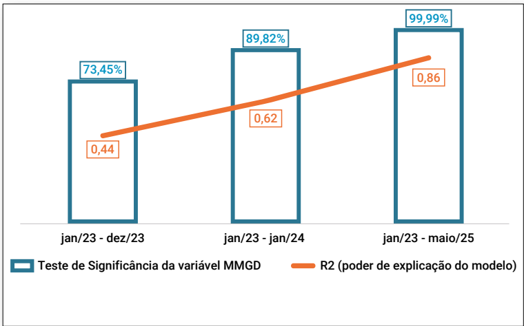
Figura 4 – Responsabilização crescente da MMGD nos volumes de curtailment
